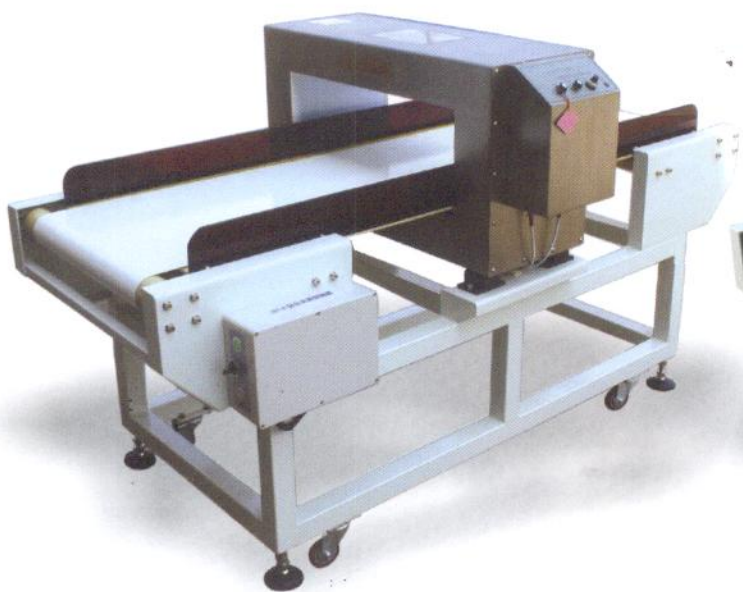
JST-A型全金属探测器(5015)
